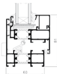
Coupe de fenêtre ouvrante
