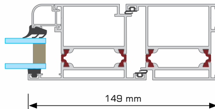
Coupe de porte
