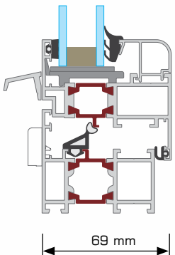
Coupe de fenêtre ouvrante
