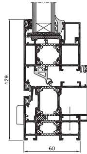
Coupe de fenêtre pivotante
