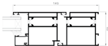
Coupe de porte
